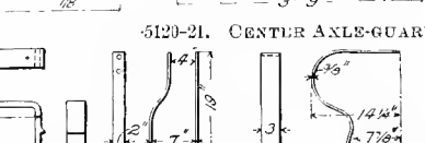
Fig. 5088. TRANSOM TIE-ROD.
